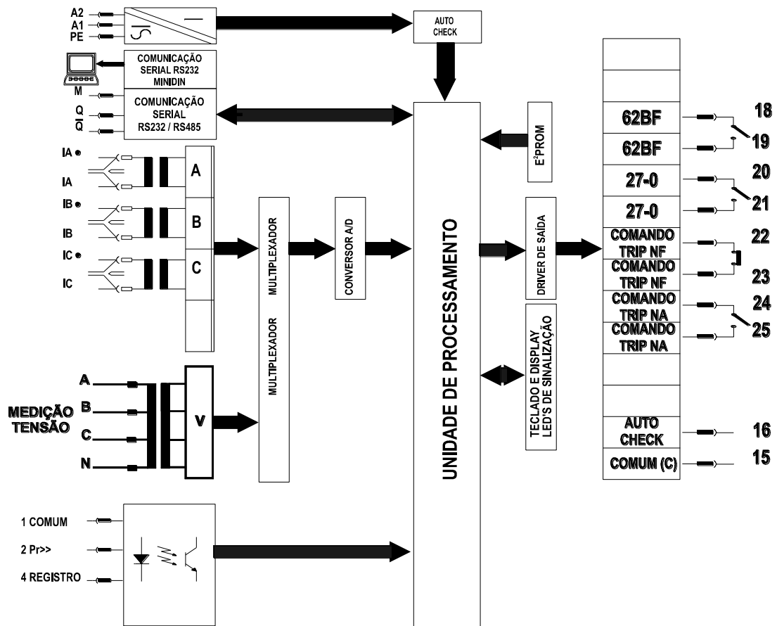
Anexo 1 _ Diagrama de blocos URPP 2405
