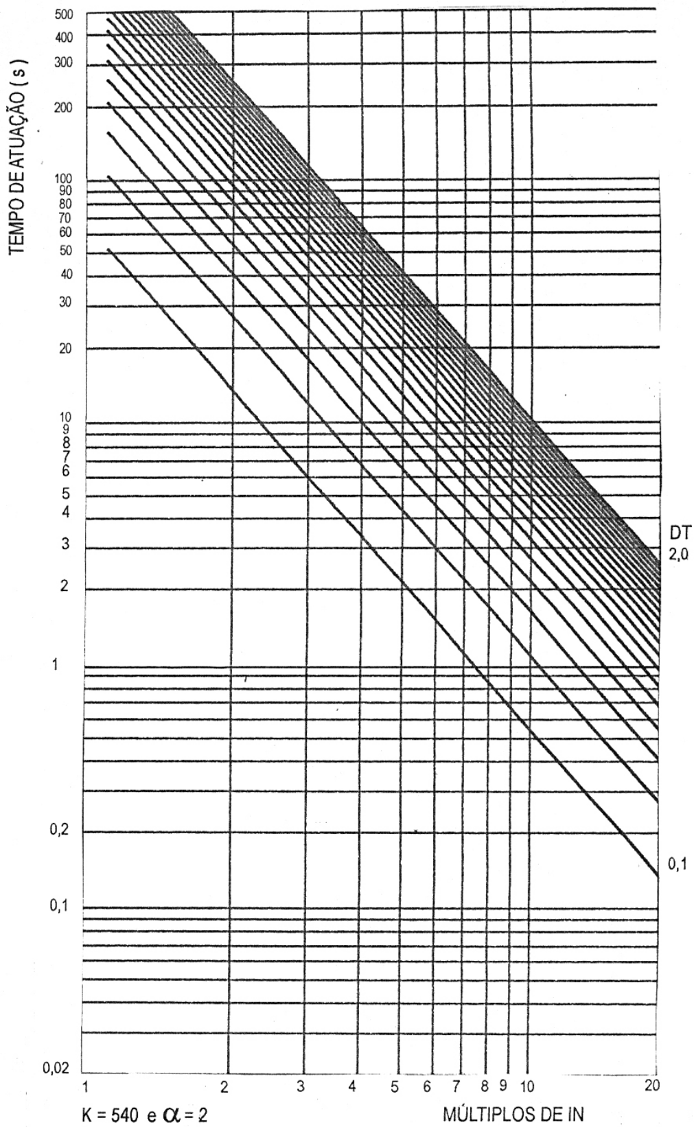
Anexo 6 – Curva I 2 T
