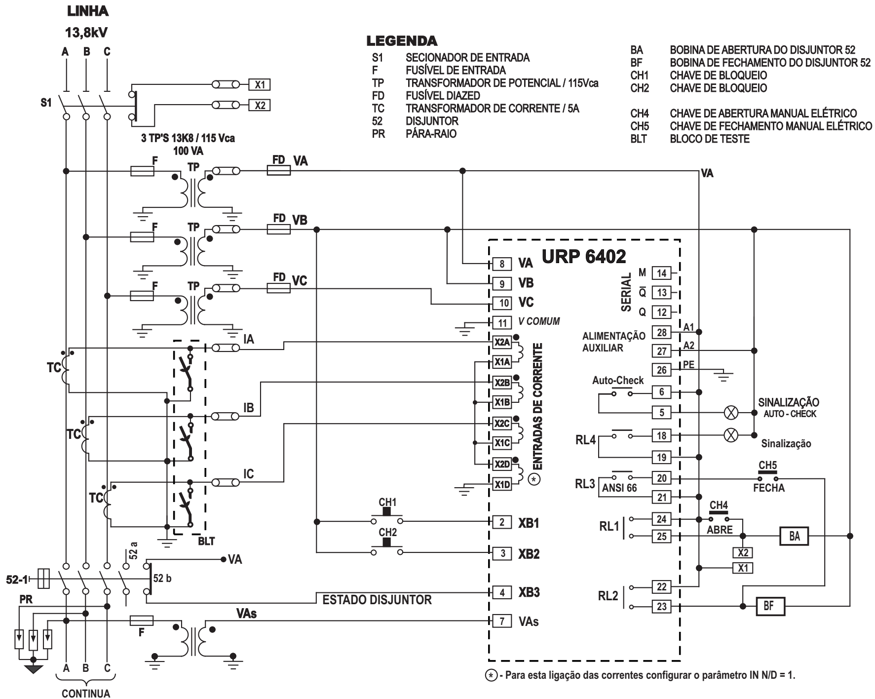
Anexo 4 C1 - Exemplo: esquema de ligação do URPS2406 com URP 6402.
