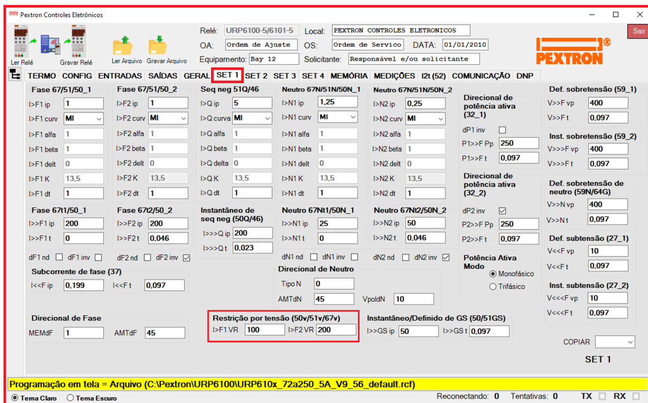
Figura 8.7: Pasta SET 1 sinalizando a unidade de sobrecorrente tempo dependente com restrição por tensão.
