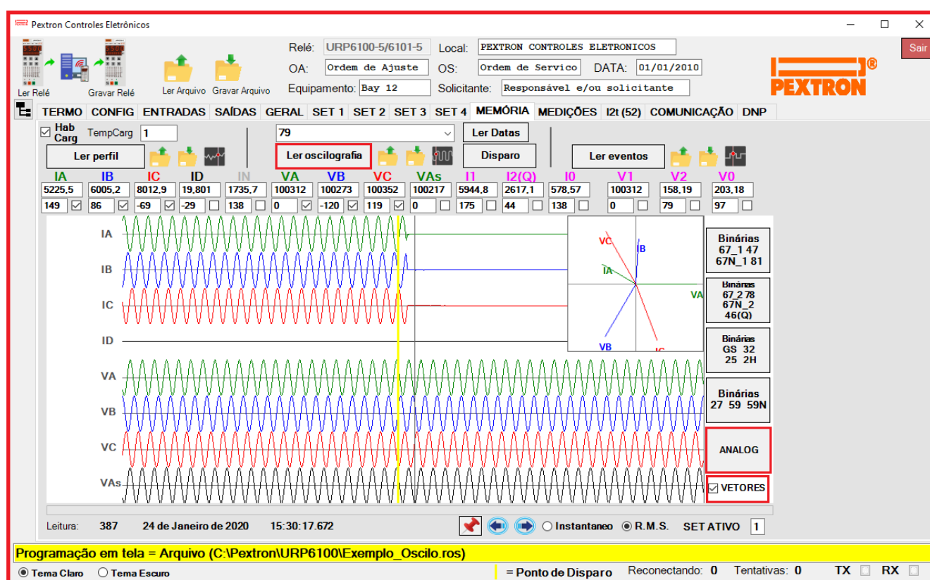
Figura 21.8: Exibição do quadro dos Fasores para o primeiro cursor
