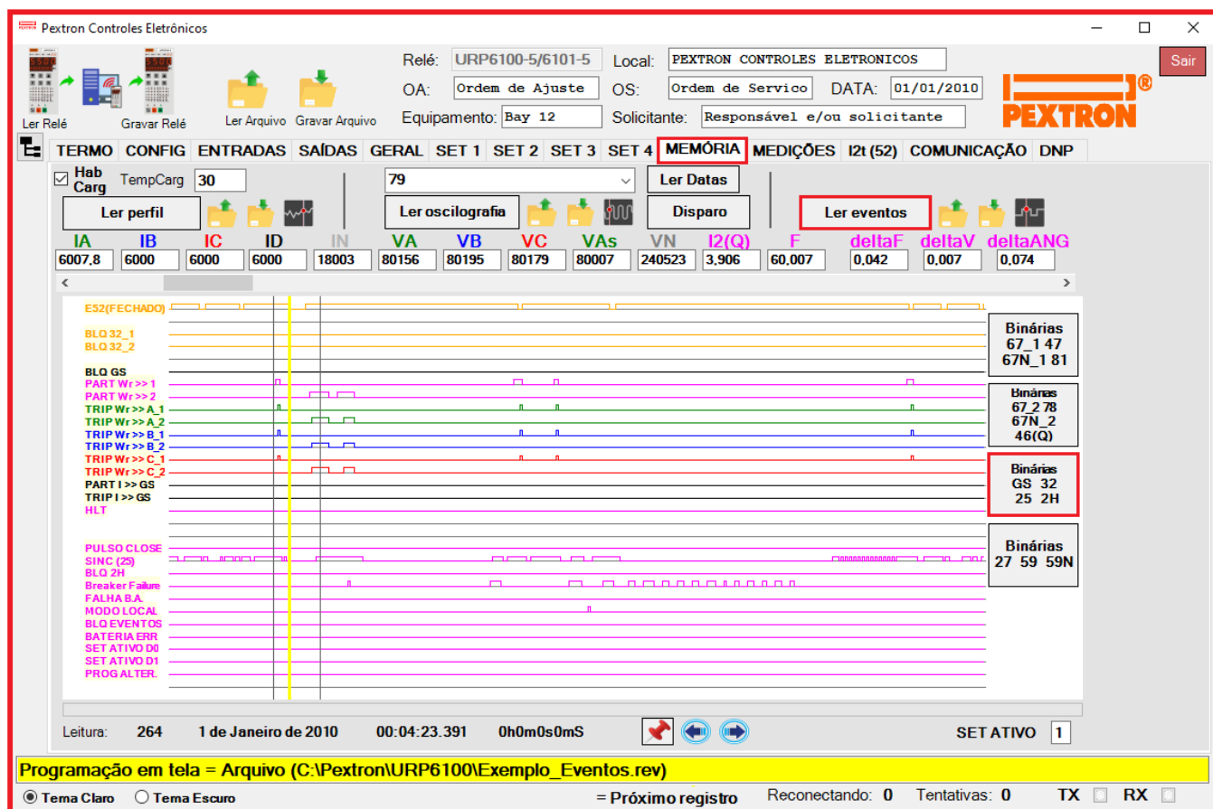
Figura 21.12: Registro de Eventos com as funções Binárias GS / 32_1 / 32_2 / 25 / 2H selecionadas.
