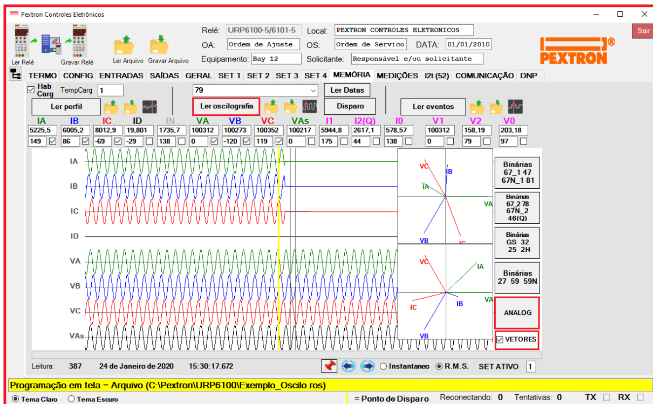
Figura 21.9: Exibição do segundo quadro dos Fasores.
