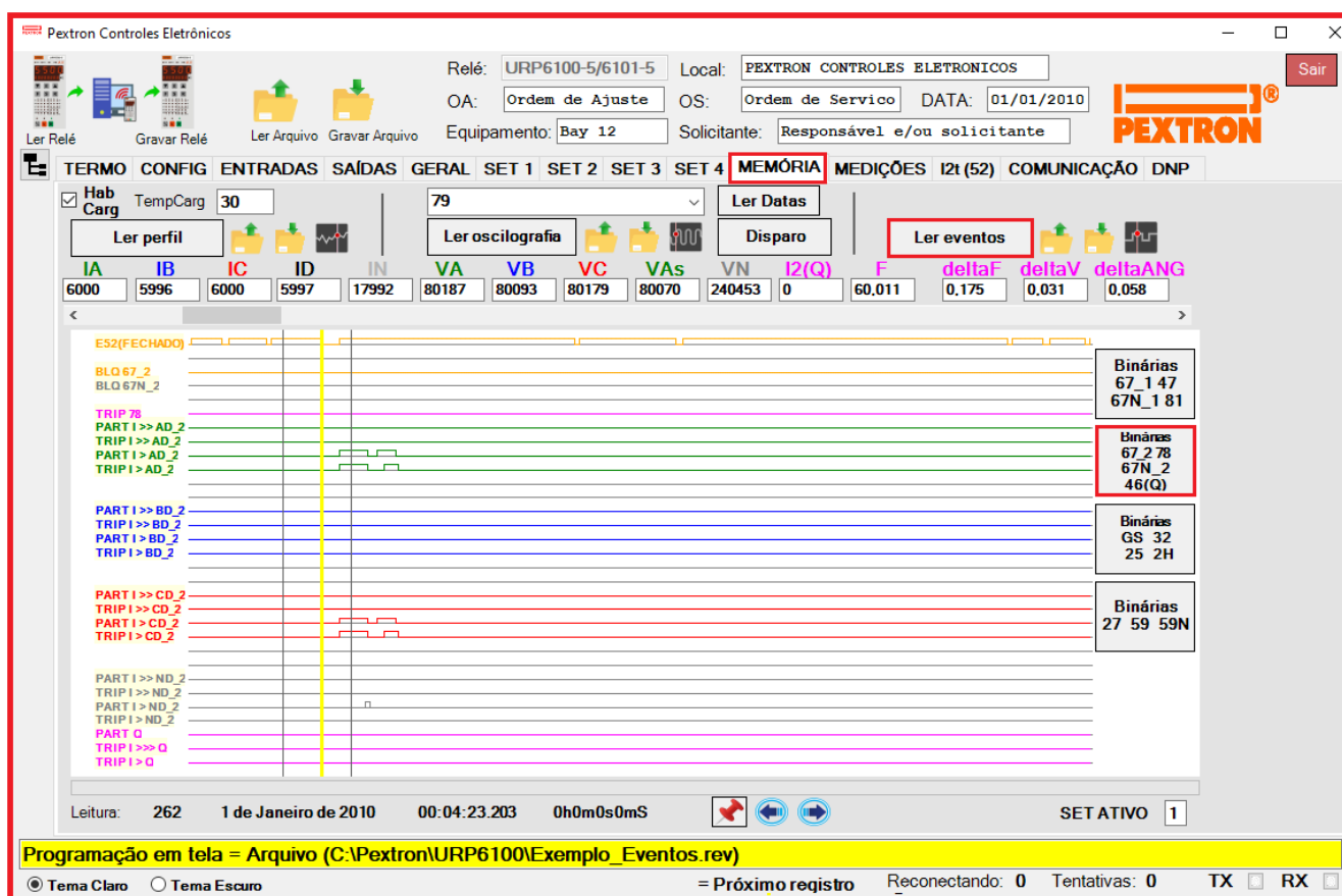
Figura 21.11: Registro de eventos nas funções binárias 67_2 / 67N_2 / 78 / 46(Q).
