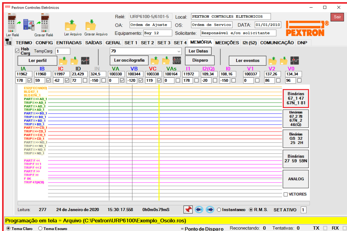
Figura 21.4: Registro de Oscilografia para exibir as funções binárias 67_1, 47, 67N_1, 81.
