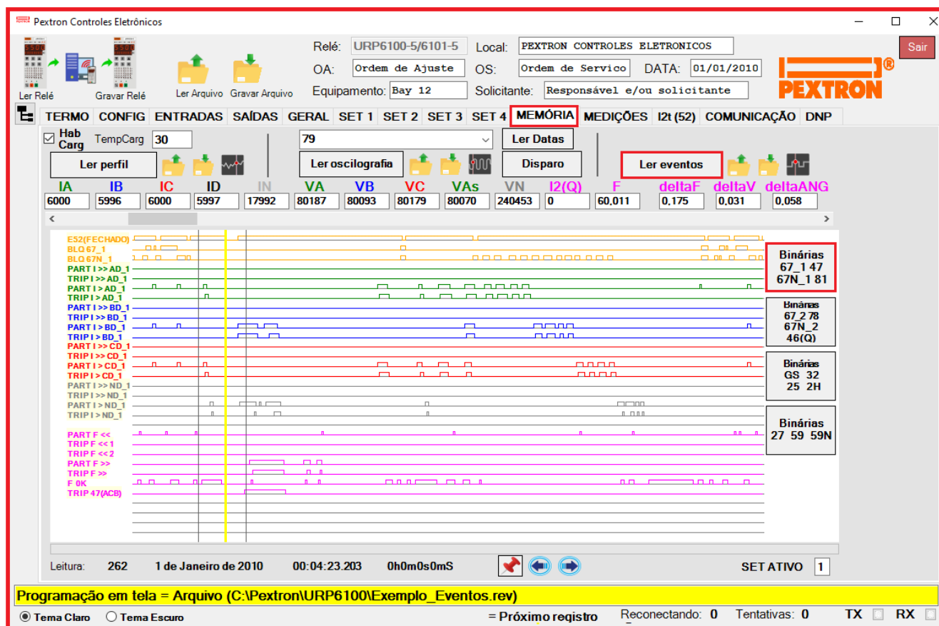
Figura 21.10: Pasta MEMÓRIA o com leitura de registro de eventos (Binárias 67_1 / 67N_1 / 47 / 81) .
