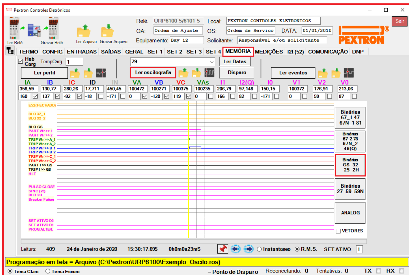
Figura 21.6: Registro de Oscilografia para exibir as binárias GS / 32_1 / 32_2 / 25 / 2H.
