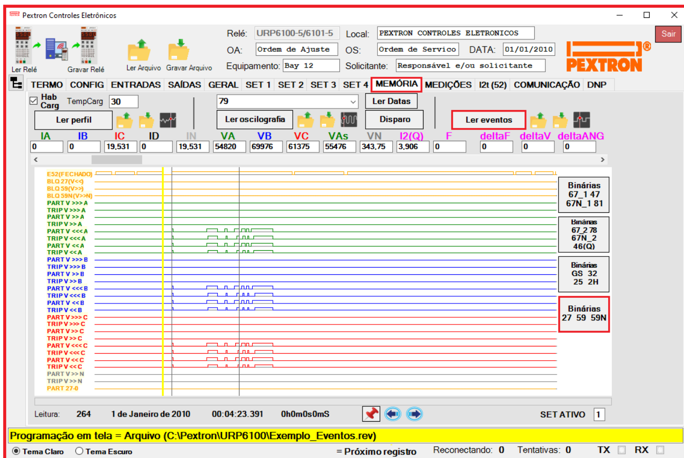
Figura 21.13: Registro de eventos nas funções binárias 27 / 59 / 59N.
