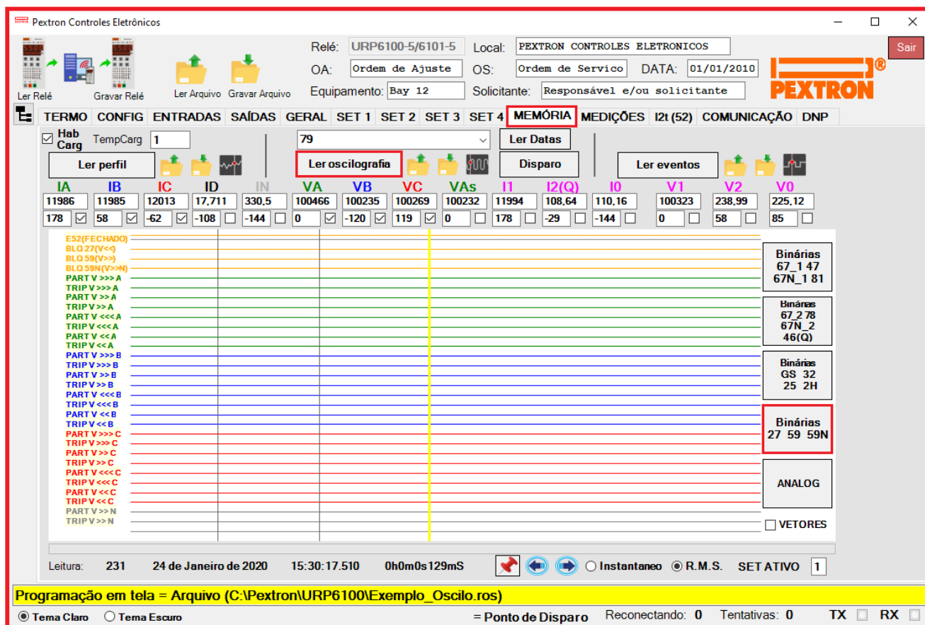
Figura 21.7: Registro de Oscilografia para exibir as binárias 27 / 59 / 59N selecionadas.
