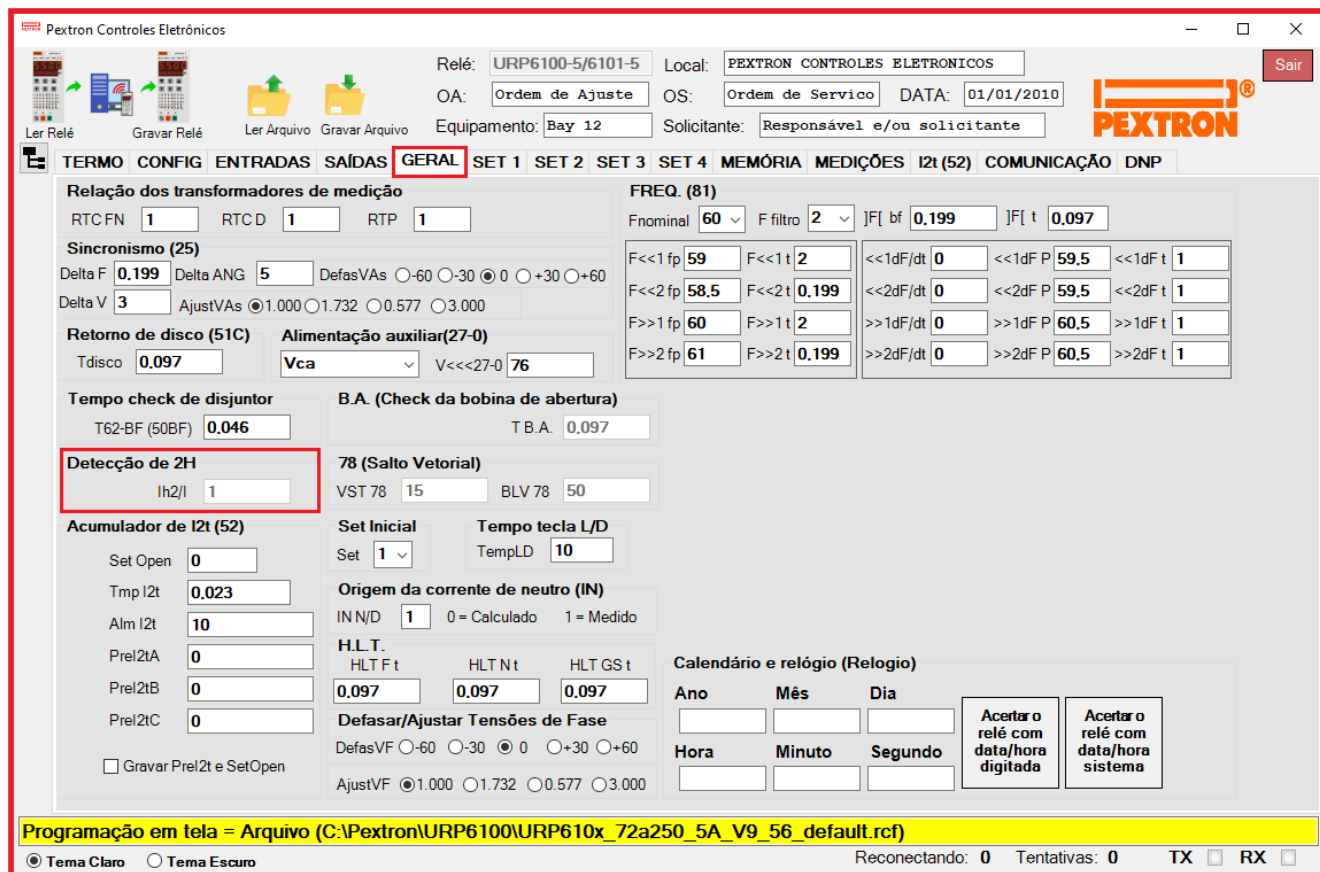
Figura 12.1: Pasta GERAL sinalizando a unidade de bloqueio por 2ª harmônica.
