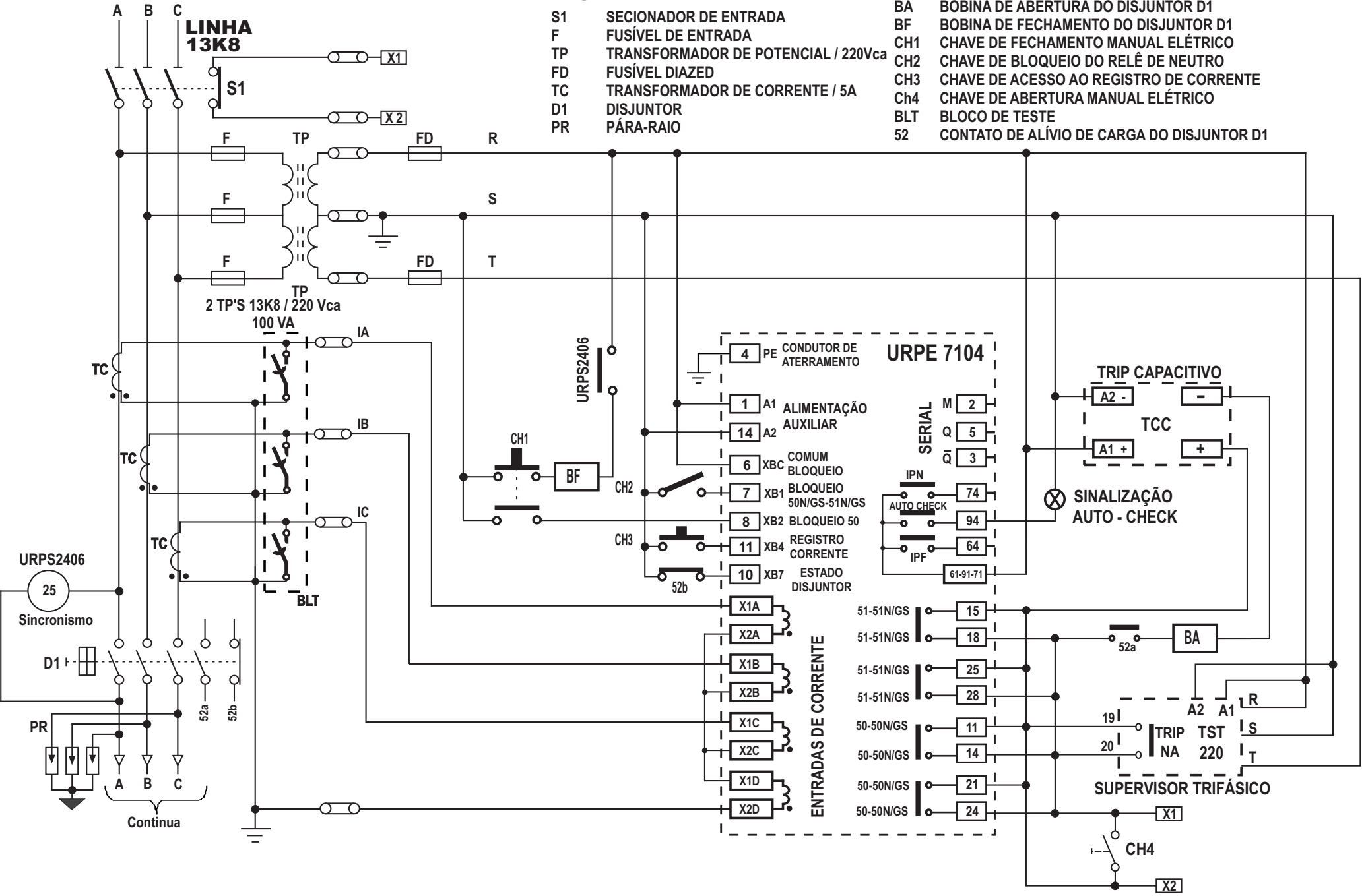
Anexo 4 B1 - Exemplo de ligação do URP610x com URPE7104.
