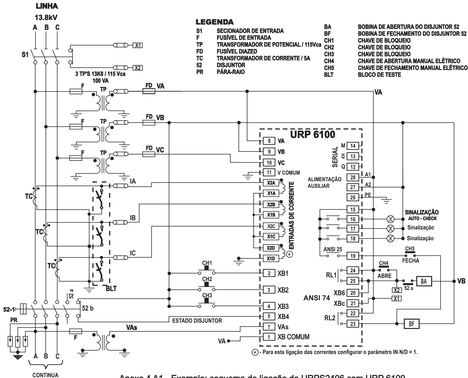
Anexo 4 A1 - Exemplo: esquema de ligação do URPS2406 com URP 6100.
