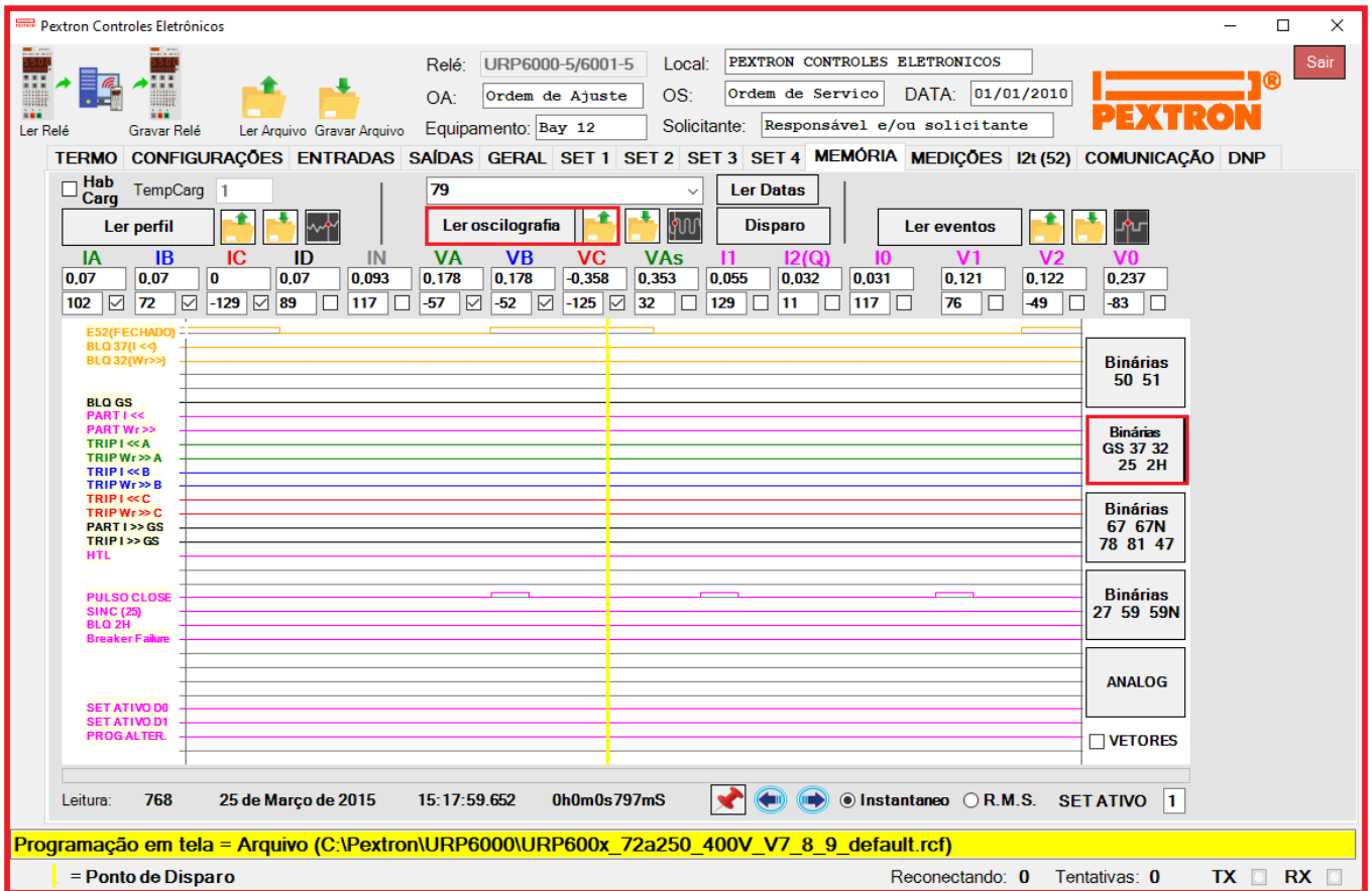
Figura 21.6: Registro de Oscilografia para exibir as binárias GS/ 37 / 32 / 25 / 2h.
