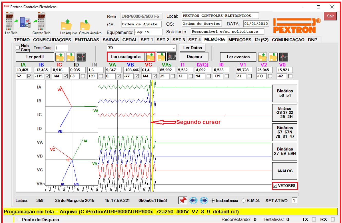
Figura 21.10: Exibição do segundo quadro dos Fasores.
