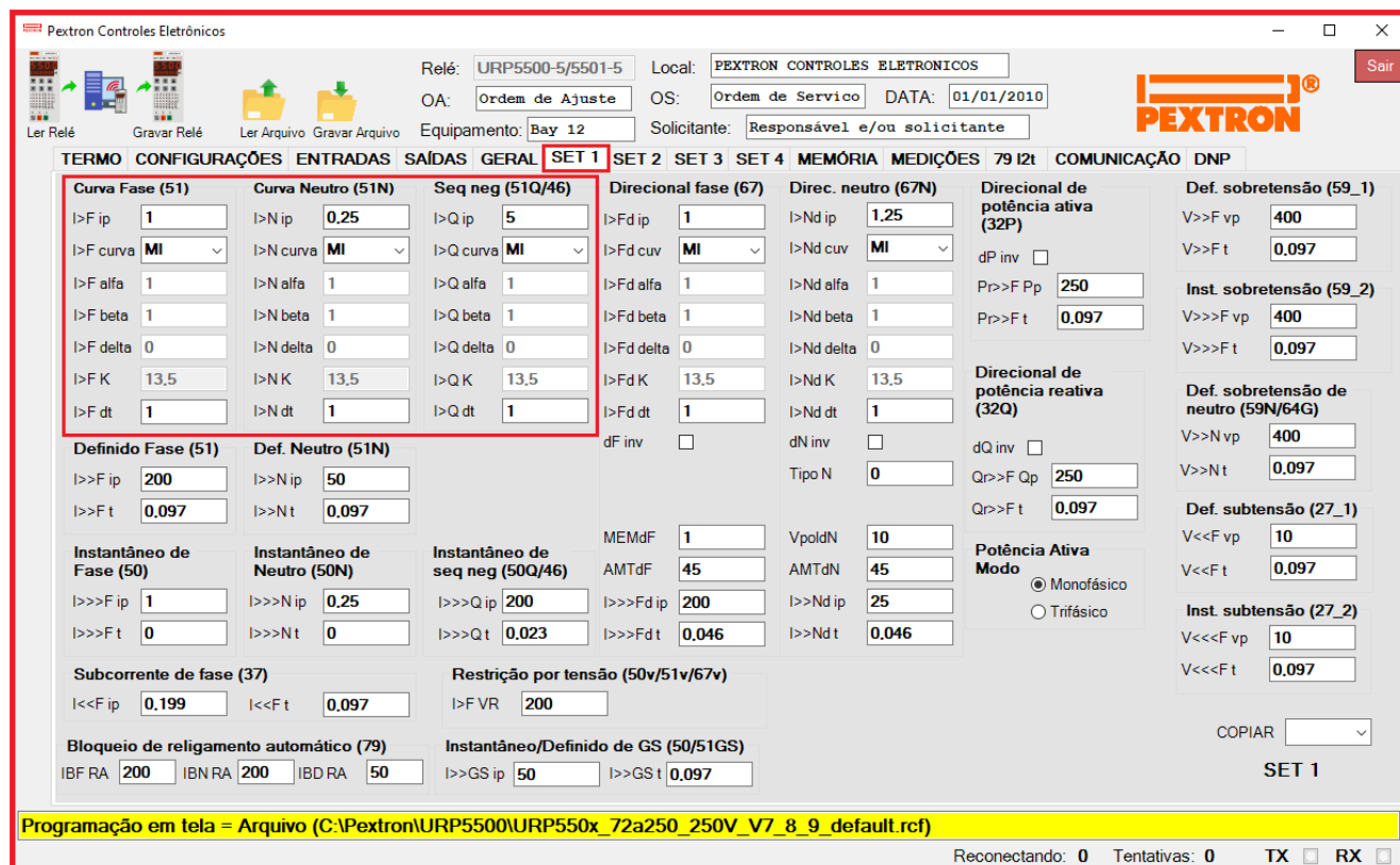
Figura 8.4: Pasta SET 1 sinalizando a unidade temporizada de tempo dependente.
