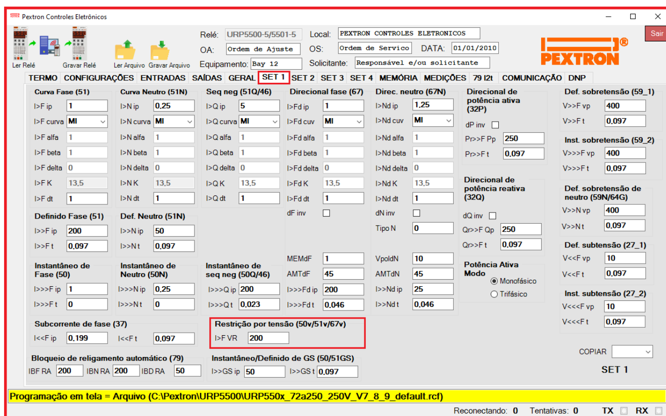
Figura 8.8: Pasta SET 1 sinalizando a unidade de sobrecorrente tempo dependente com restrição por tensão.
