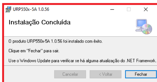
Figura 3.19: Concluir instalação.
