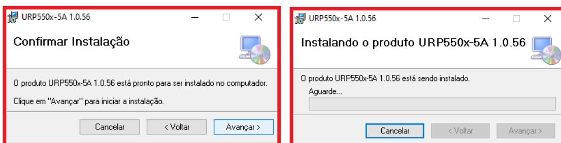
Figura 3.18: Confirmar instalação.
