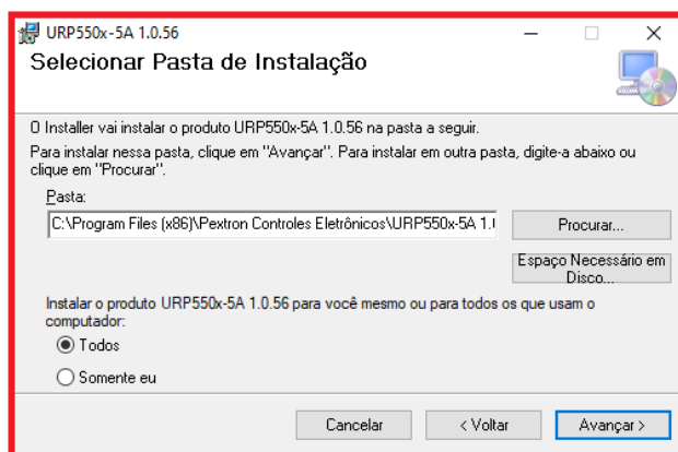
Figura 3.17: Selecionar pasta.
