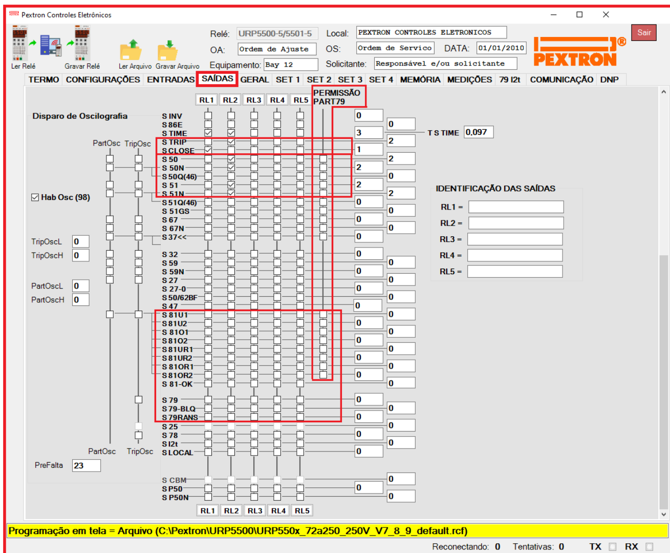
Figura 15.3: Pasta SAÍDAS do programa aplicativo sinalizado com permissão da unidade de religamento automático.
