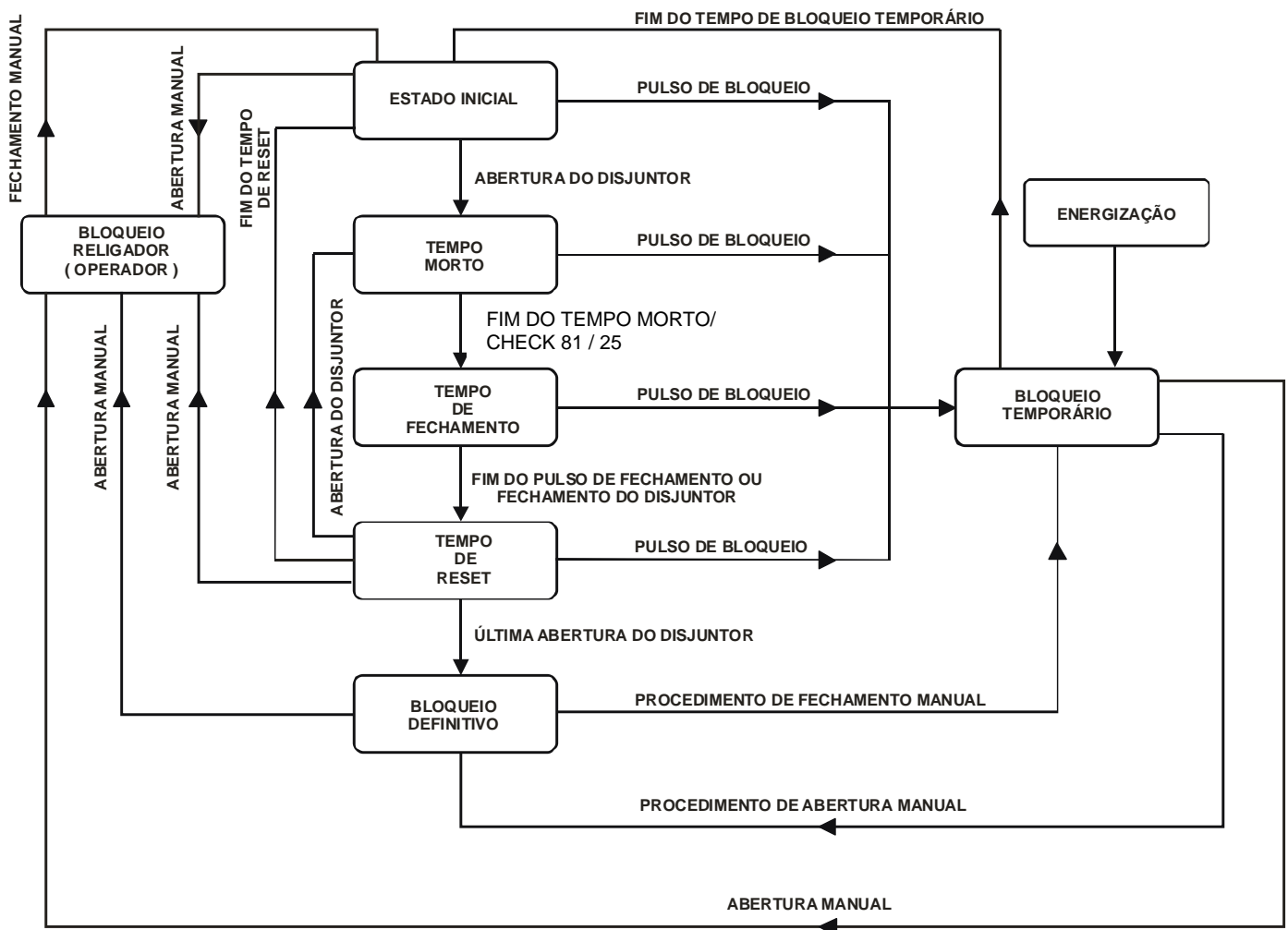
Figura 15.4 : Diagrama de blocos dos estados de funcionamento da unidade de religamento.
