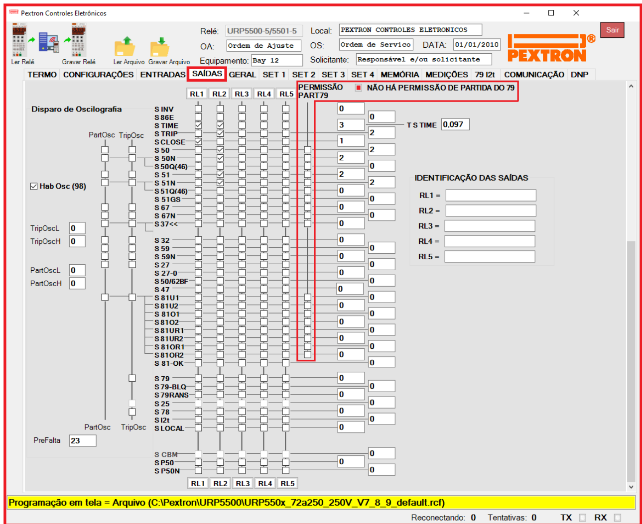
Figura 15.2: Pasta SAÍDAS do programa aplicativo sinalizado sem permissão da unidade de religamento automático.
