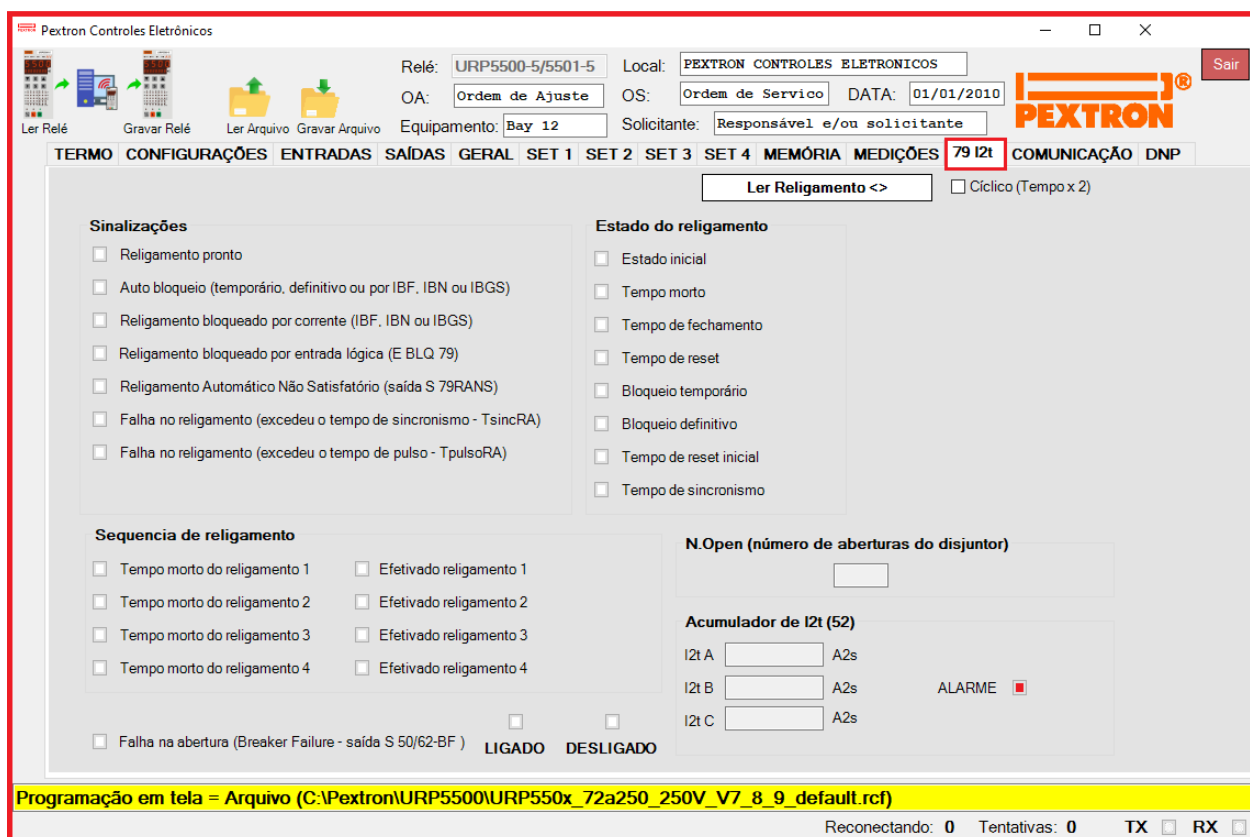
Figura 15.6: Pasta 79 I2t sinalização das condições de operação da unidade de religamento automático.
