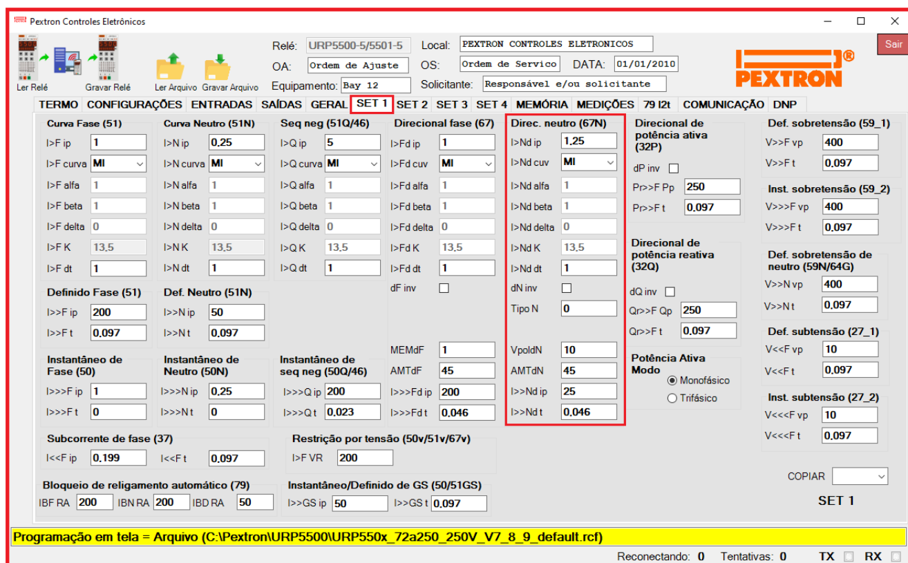
Figura 10.4: Pasta SET 1 sinalizado com os parâmetros da unidade de sobrecorrente direcional de neutro.
