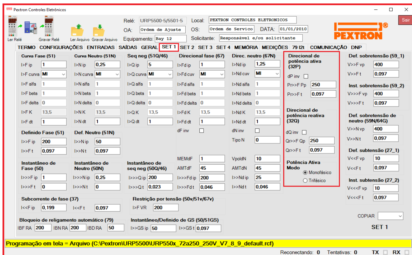
Figura 10.9: Pasta SET 1 sinalizado com os parâmetros da unidade direcional de potência.
