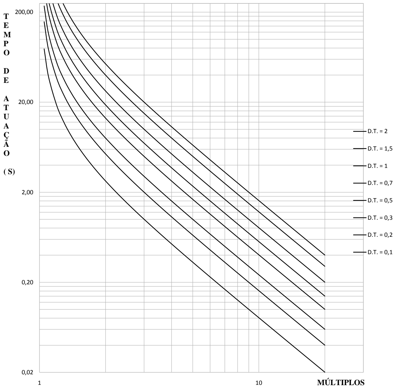
CURVA EXTREMAMENTE INVERSA K = 80 α = 2
