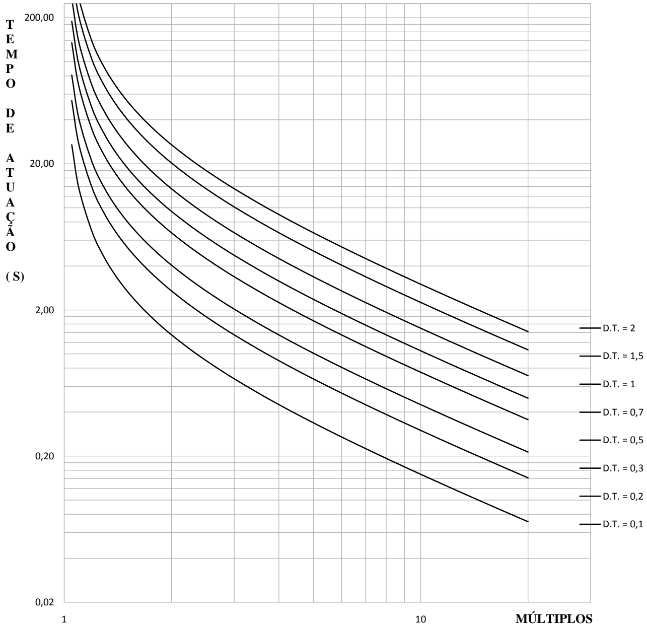
CURVA MUITO INVERSA K = 13,5 \alpha = 1
