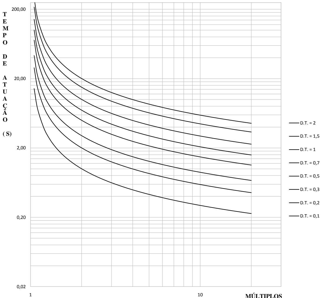
CURVA NORMALMENTE INVERSA K = 0,14 α = 0,02
