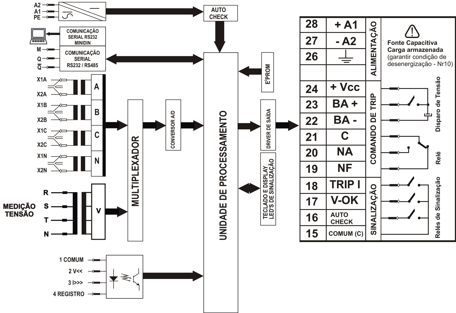
Anexo 7 _ Diagrama de blocos URP1439T
