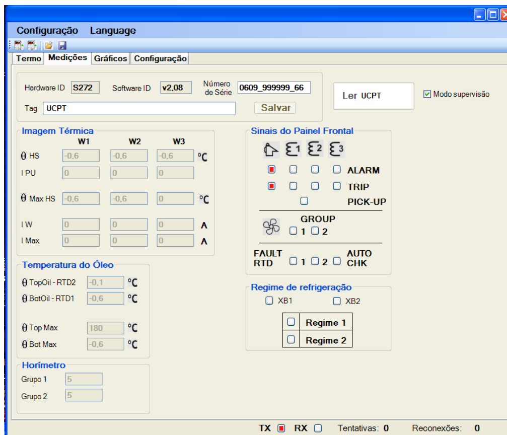
Figura 17: Tela inicial do software de parametrização e acesso a memória de massa.
