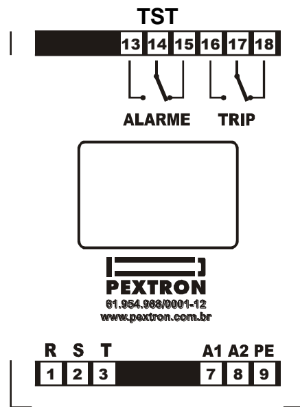
Figura 3: Identificação de bornes TST.
