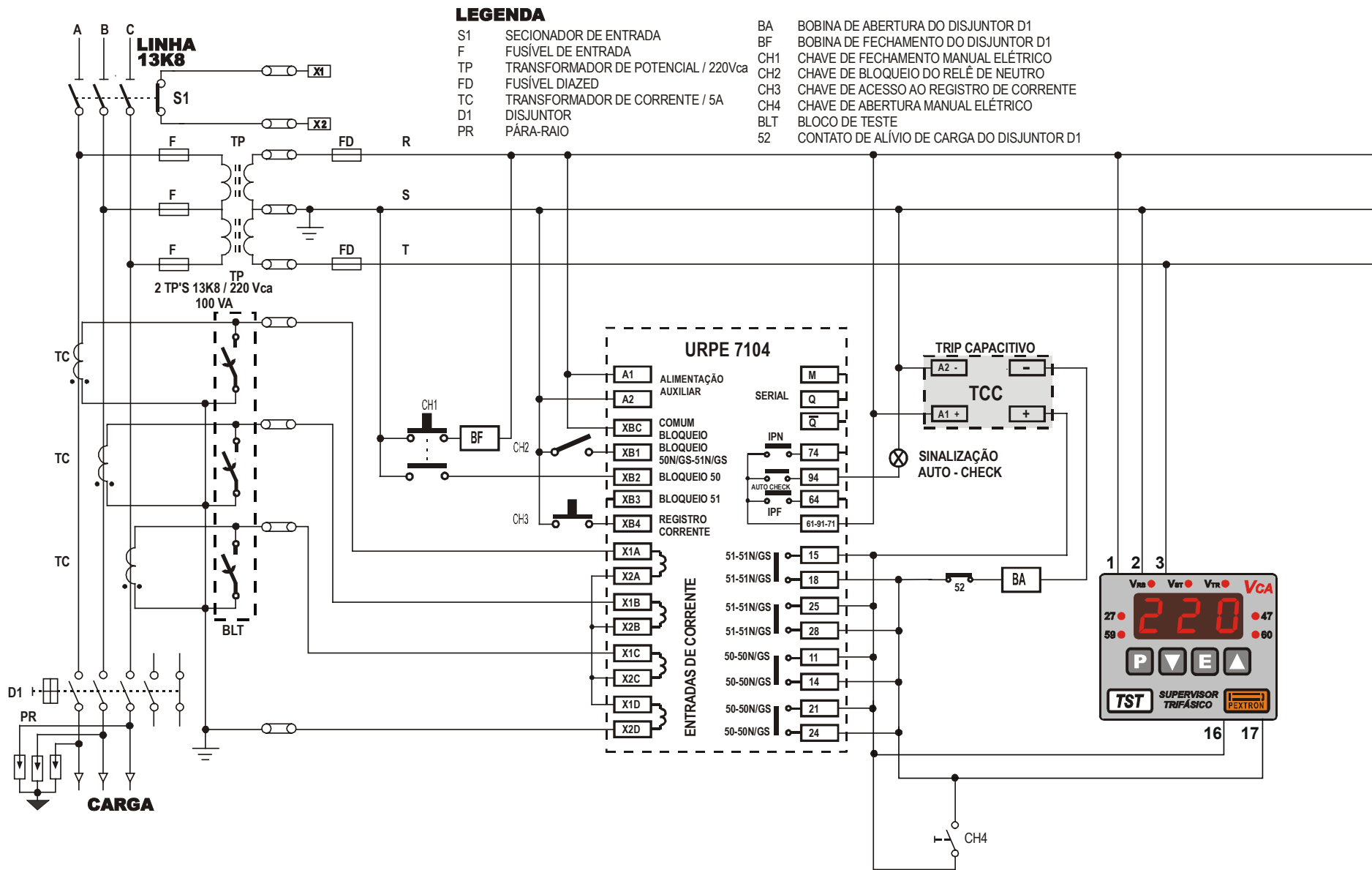
Anexo 1 : Esquema de ligação TST ( alimentação auxiliar conjugada e operação NA normal ) na cabine primária com relé URPE7104.
